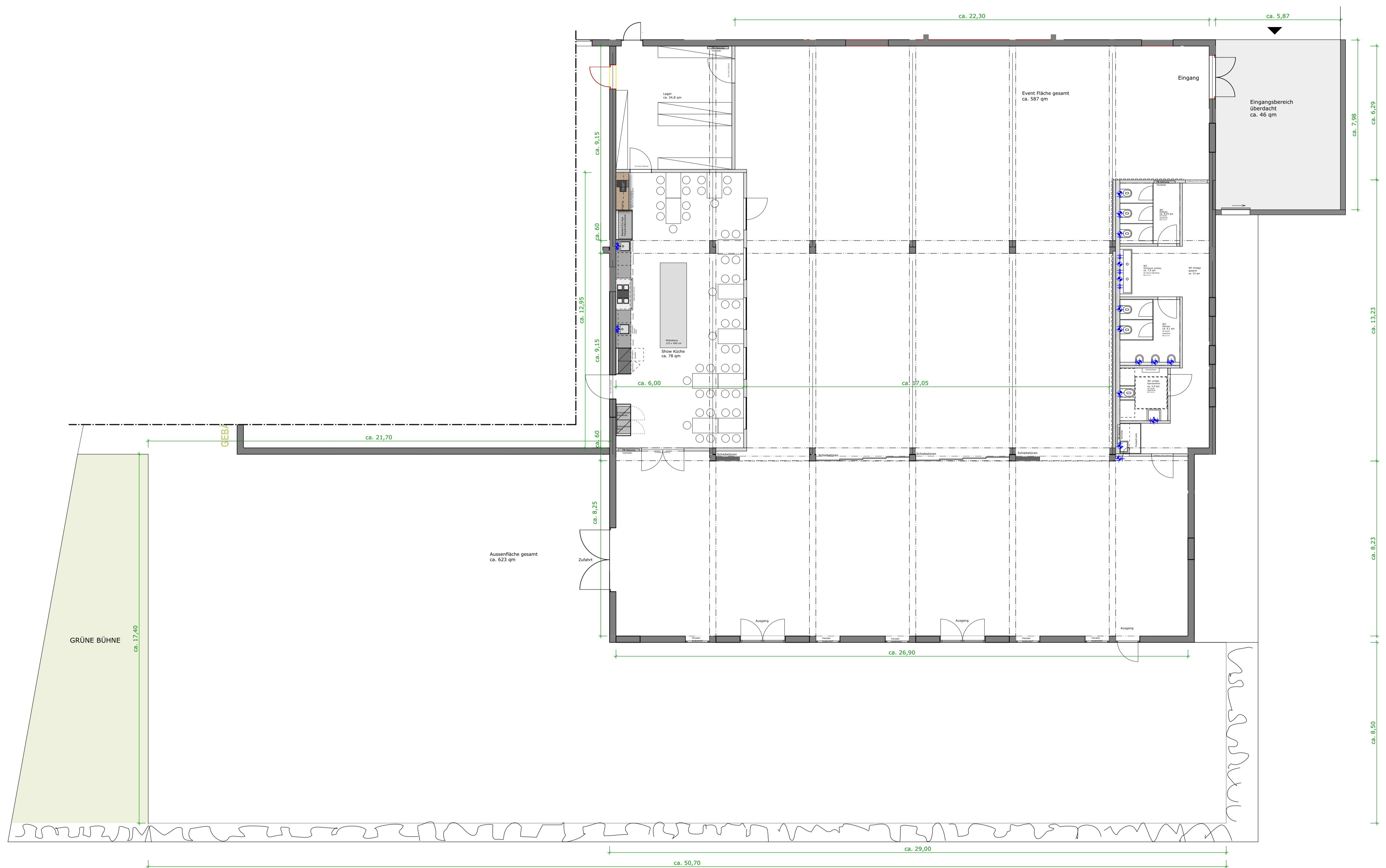
N4 Eventlocation Grundriss Maßstab 1:100
